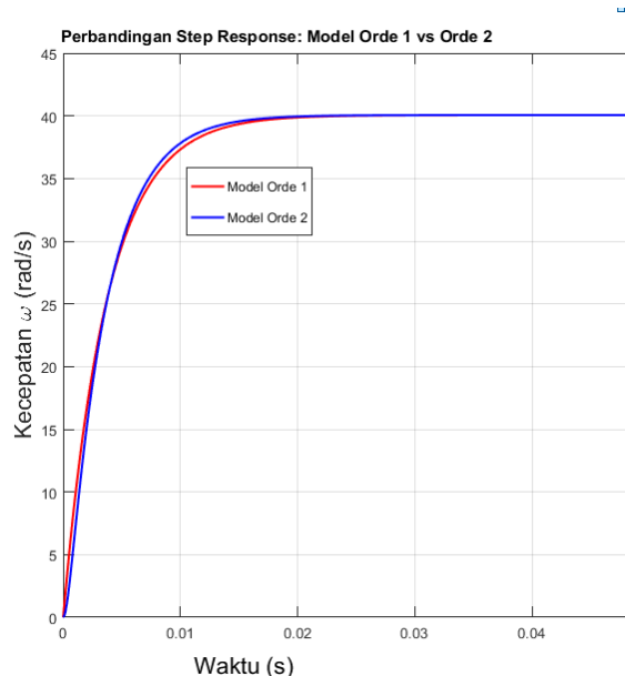
Gambar 1. Perbandingan kurva respon kecepatan motor DC Maxon DCX 35 L terhadap input step 24 V antara model orde satu (merah) dan model orde dua (biru). Model orde dua menunjukkan performa dinamis yang lebih cepat dan stabil, dengan error steady state lebih kecil.
